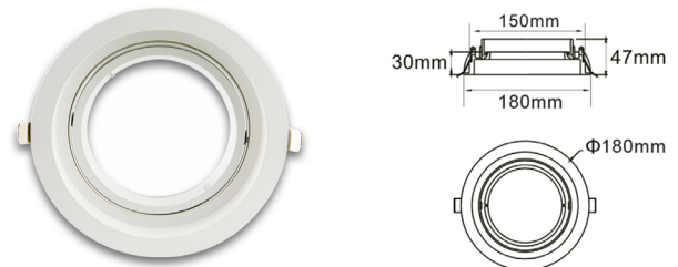
112579 | AR 111, rond, platencastré, pivotant
